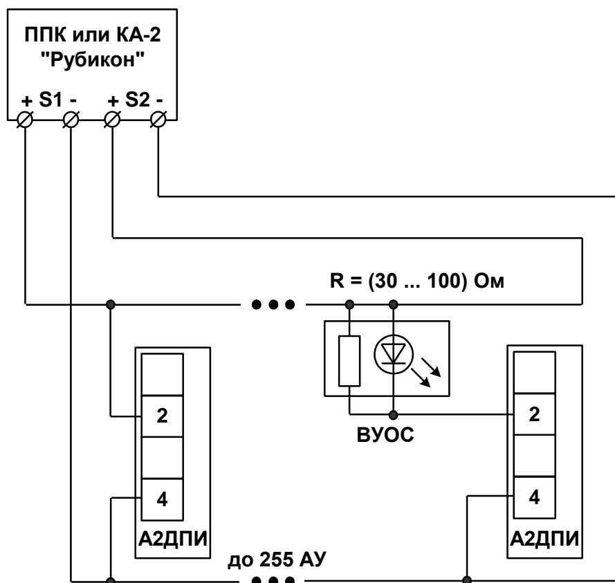
Рис. 4 Подключение А2ДПИ-052 (подключается в АШ ППК или КА-2)
