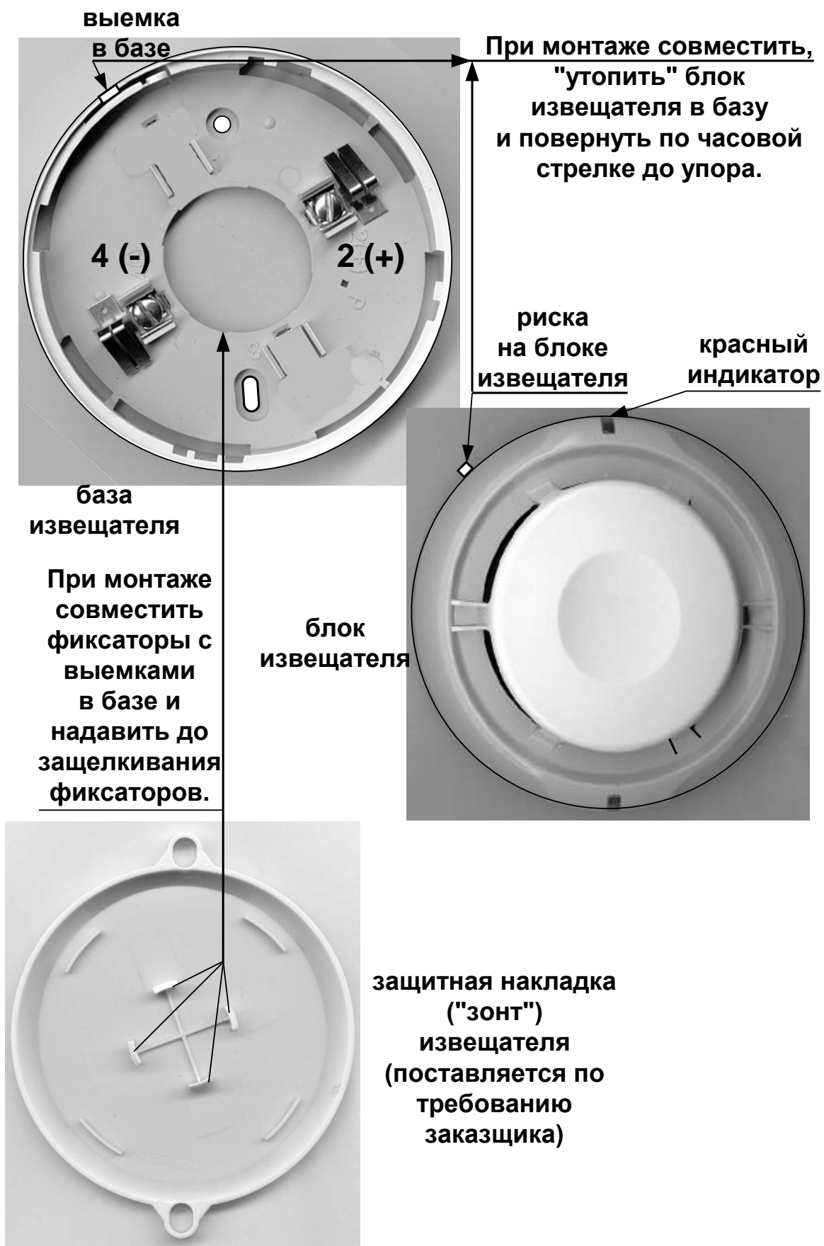
Рис. 1 А2ДПИ-052 «Рубикон» (база, блок извещателя, "зонт")
