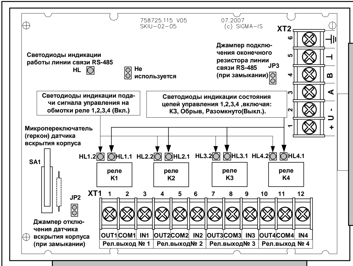
Рис. 1 Внешний вид SKIU без крышки корпуса (исполнение IP20)
