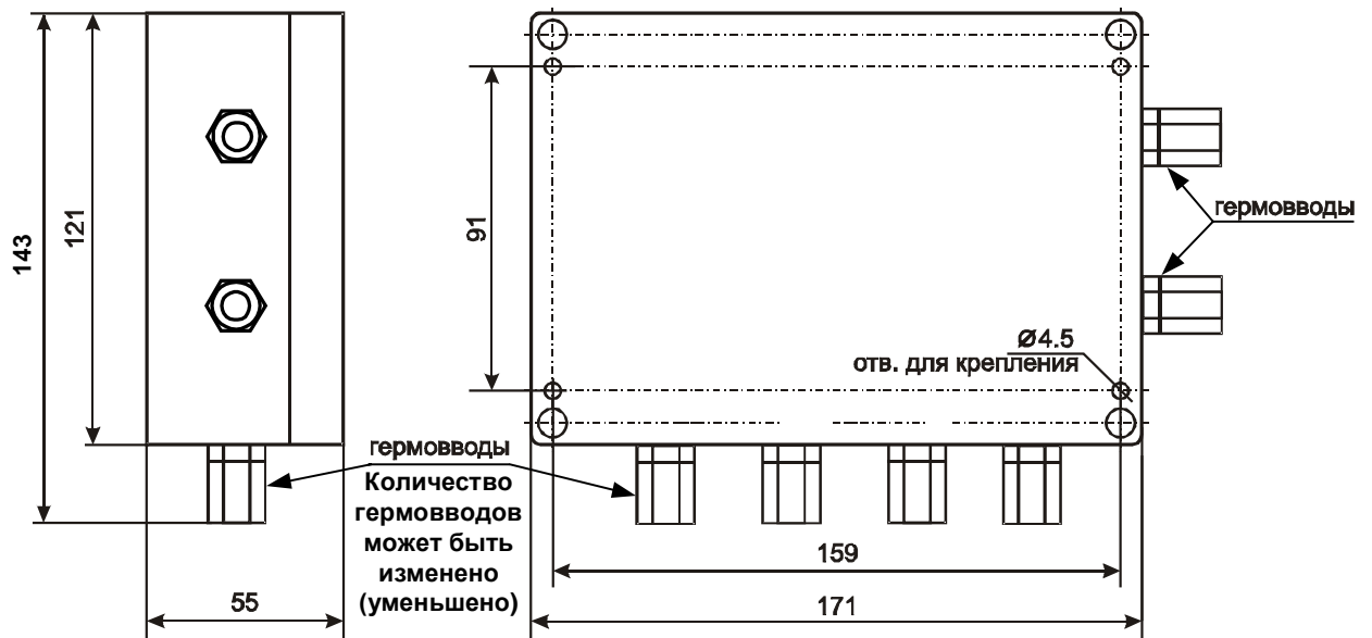
Рис. 5 Габаритные и присоединительные размеры (исполнение IP65)
